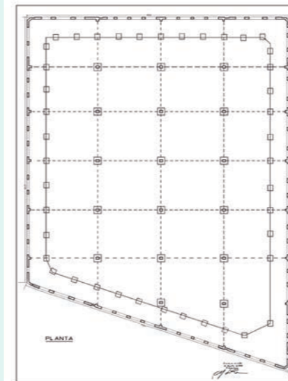
Planta do proxecto da fábrica Alfageme. Manuel Gómez Román, 1928 (Arquivo Municipal de Vigo).
