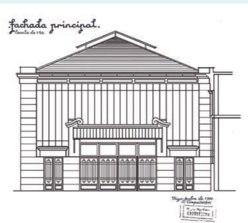
Proxecto de ampliación da fábrica Alfageme. Fachada principal. Manuel Gómez Román 1939. (Arquivo Municipal de Vigo).
